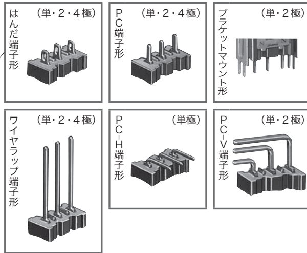
端子部形状
