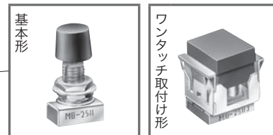
操作部形状
